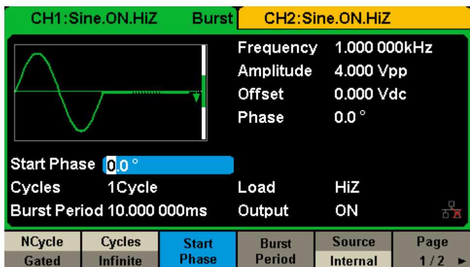
Рис. 9-31 Окно генератора в пакетном режиме/ BURST
