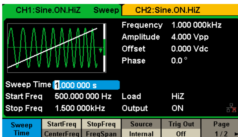
Рис. 9-30 Окно генератора в режиме ГКЧ/SWEEP
