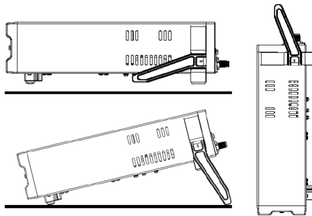
Рис. 6.1 Регулировка положения ручки:
