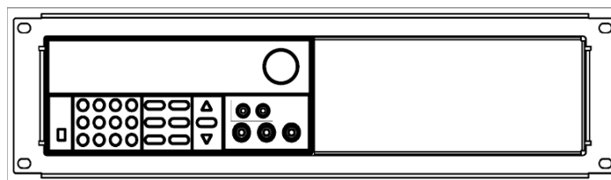
Пример установки одного ИП в панель IT-E151 для монтажа стойку
