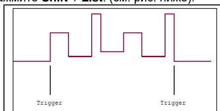
Рис. 7.2. Все шаги профиля последовательно следуют друг за другом с момента старта до остановки.
