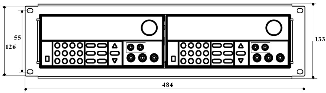
Пример установки двух ИП в ряд в панель IT-E151 для монтажа стойку
