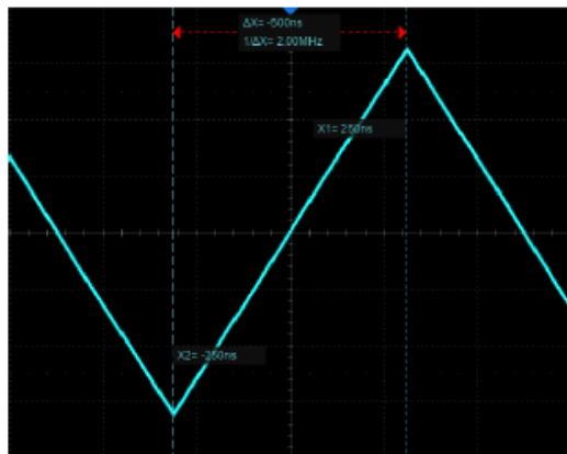
X-курсоры (временной домен)
