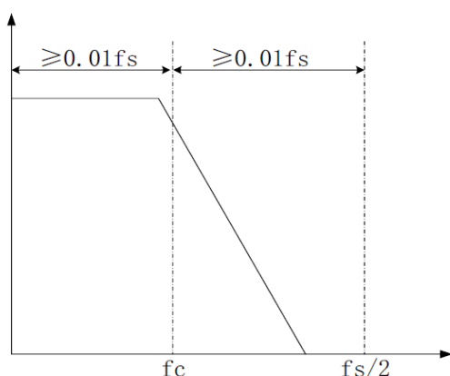
НЧ-фильтр
