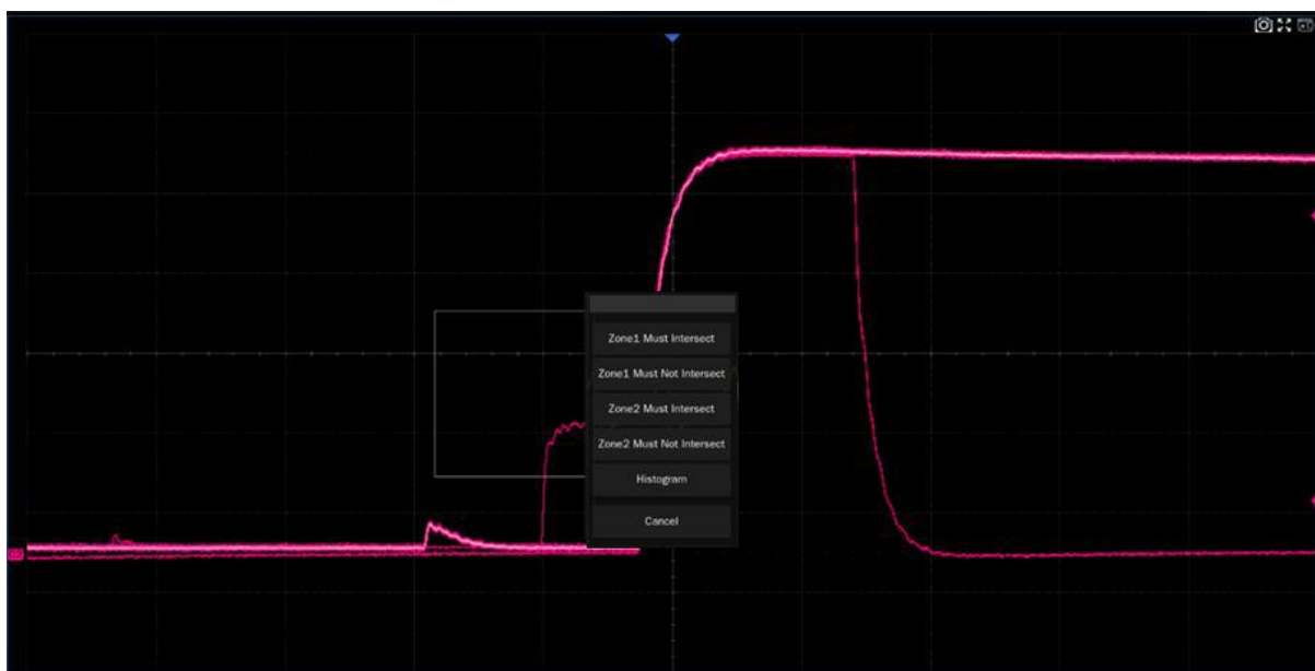
Рис. 18-4 Пример выделения области синхронизации
