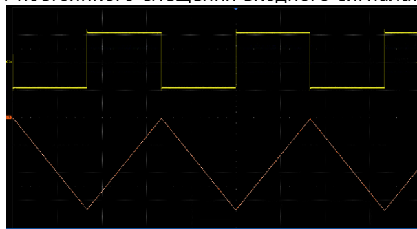
Результат интегрирования меандра с компенсацией смещения
