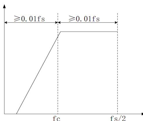
ВЧ-фильтр
