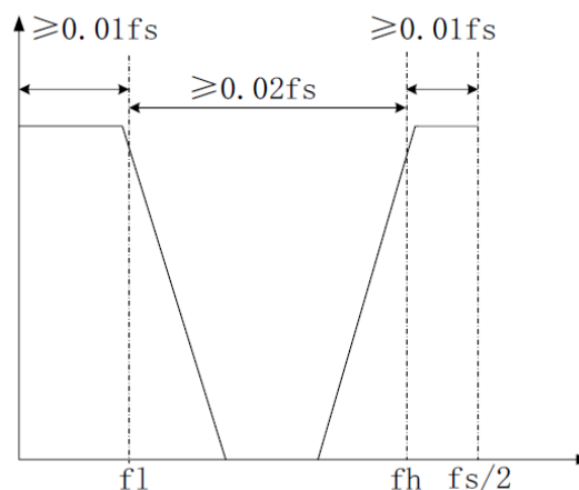
Режекторный фильтр
