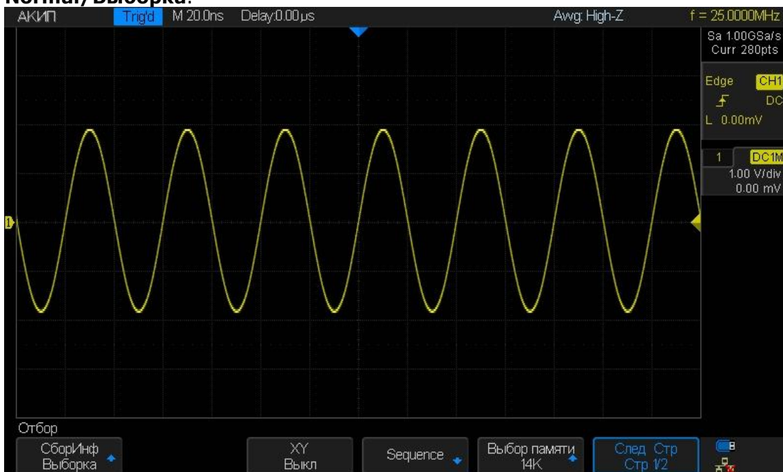
Рис. 10-4 Режим стандартной выборки
