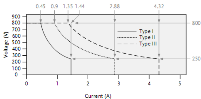
Рабочая область выходных параметров серии PSW7 250 В
