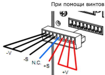
Локальное подключение обратной связи
