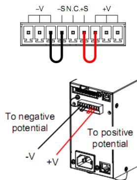
Локальное подключение обратной связи
