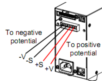
Удаленное подключение обратной связи
