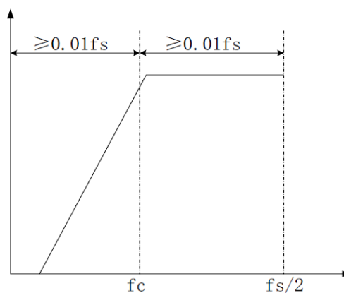
НЧ-фильтр
