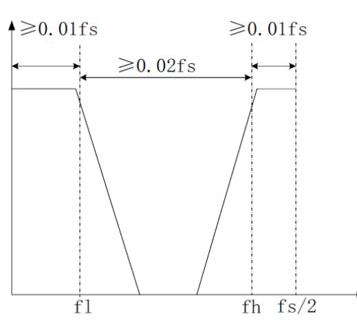
Режекторный фильтр
