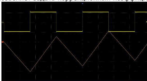
Результат интегрирования сигнала прямоугольной формы без смещения
