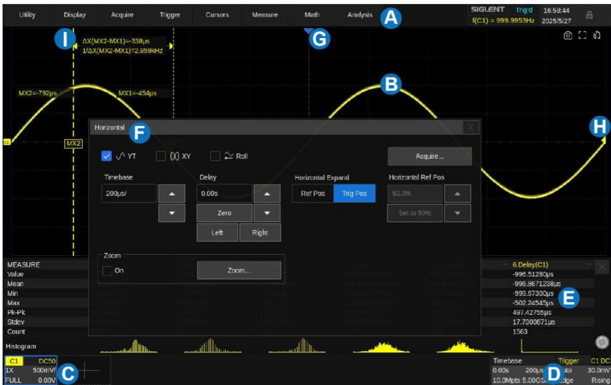
Рис. 10-1 Окно осциллографа сери АК ИП-4157
