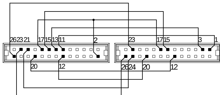
Главное устройство Подчиненное устройство 1
