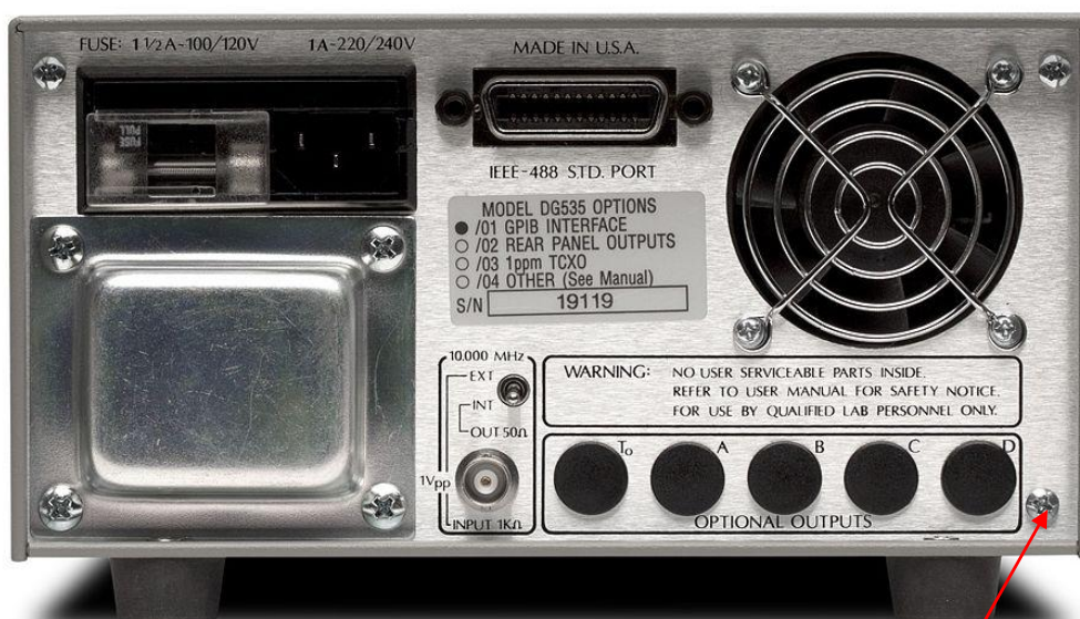
Рисунок 2 - Общий вид
