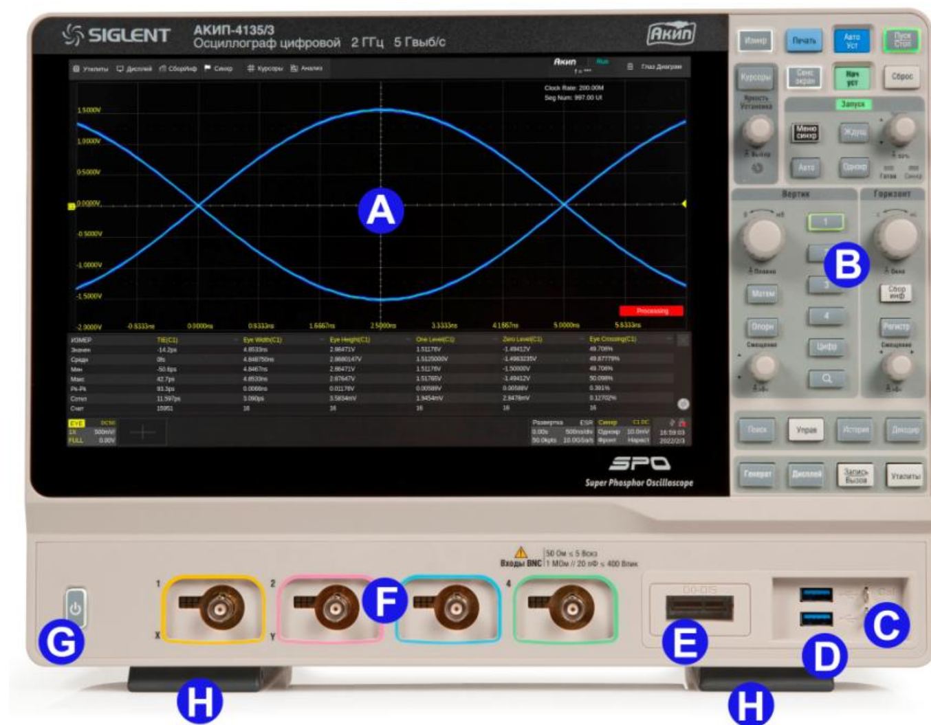
Рис. 9-1 Передняя панель осциллографов серии АКИП-4135
