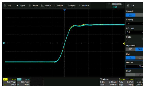
После выравнивания
