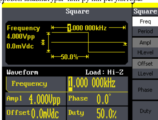
Рис. 9-5 Режим формирования сигнала прямоугольной формы, активен пункт меню Duty/Коэффициент заполнения
