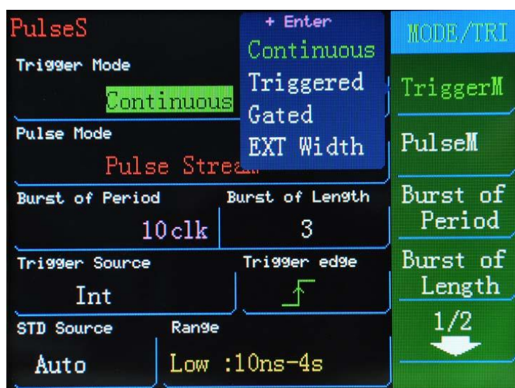
Рис.5 Экранное меню
