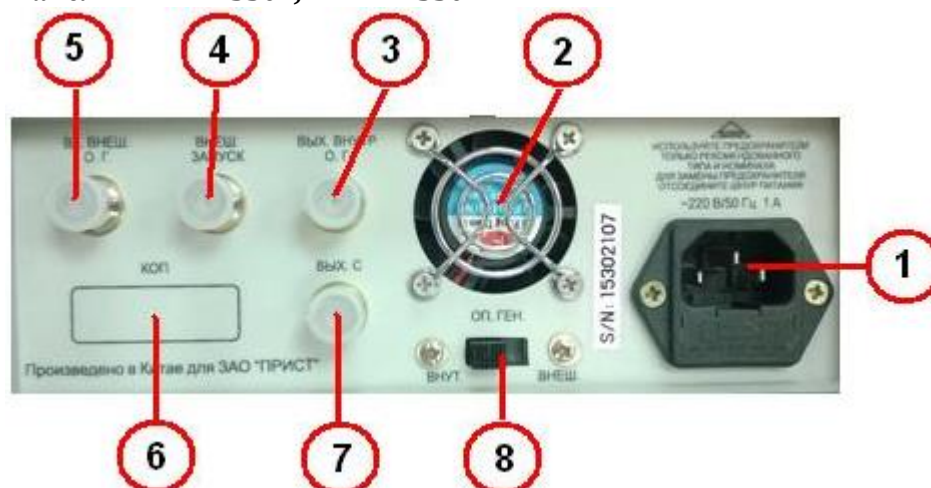
Рис.2 Задняя панель АКИП-3302
