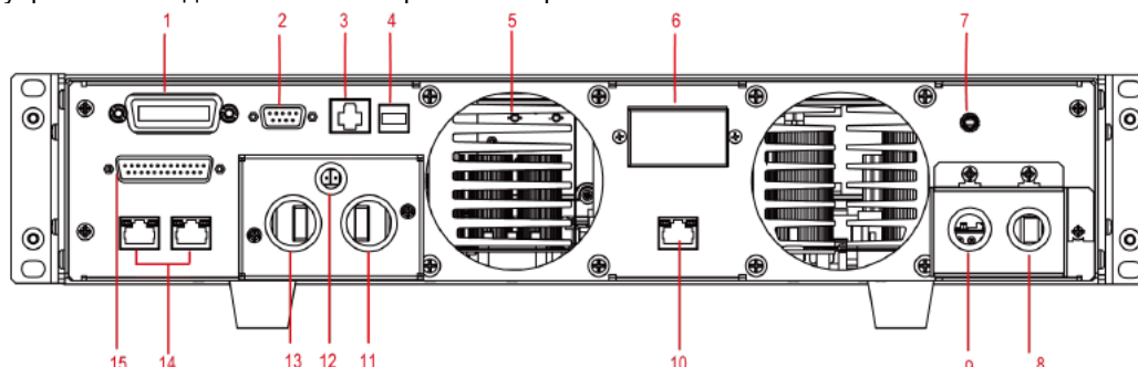
Рис. 5.2. Задняя панель
