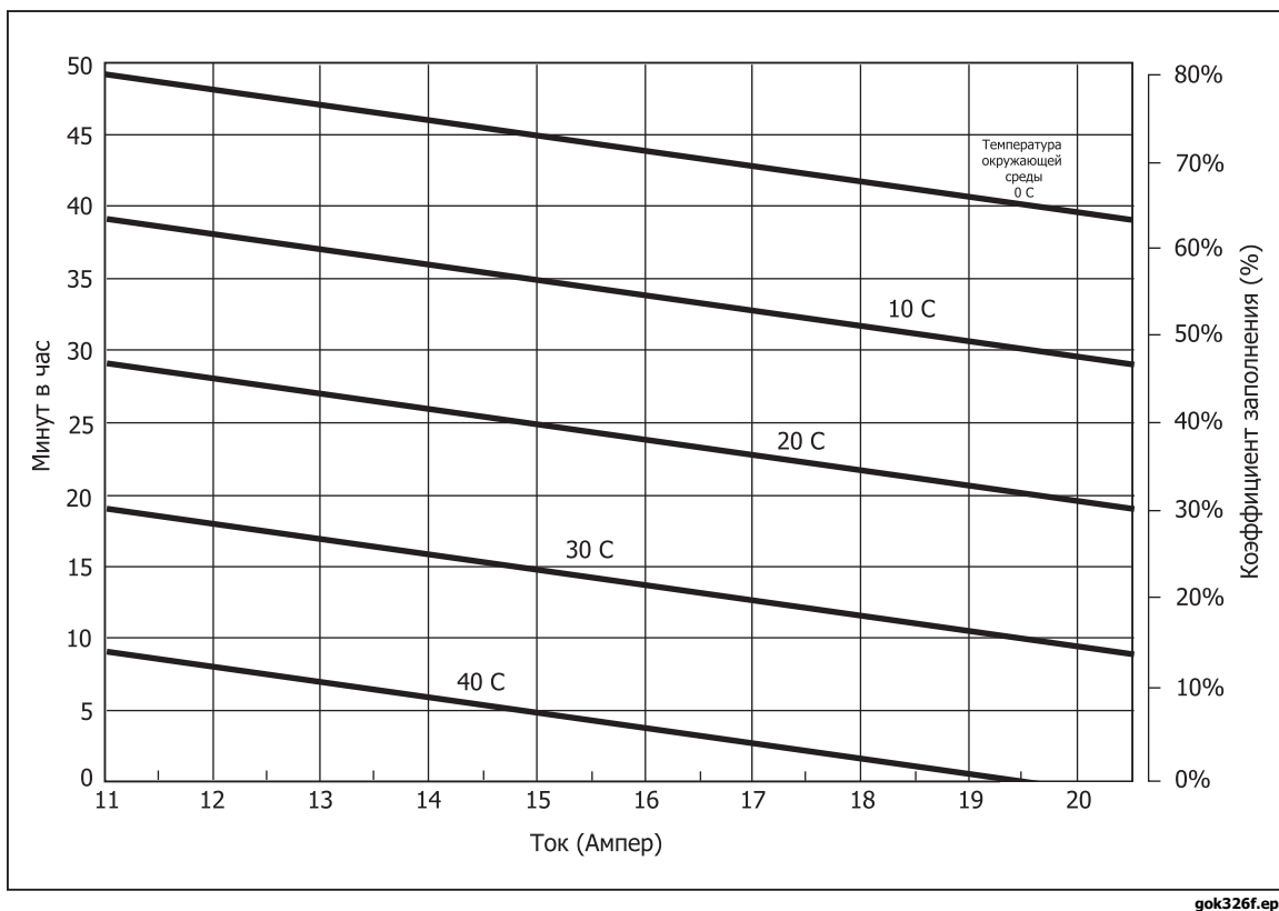
Рис. 1-3. Допустимая продолжительность работы с током более 11 А
