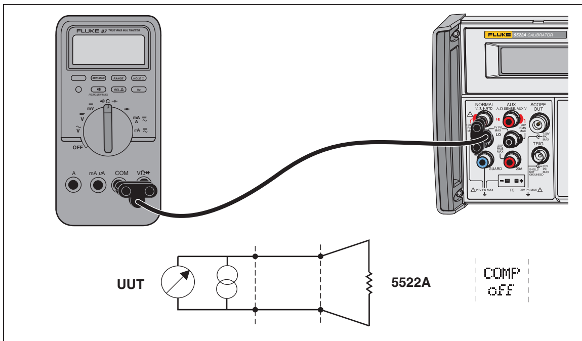
Рисунок 4-4. Подключение испытываемого устройства: Сопротивление (без компенсации) gjh016.eps
