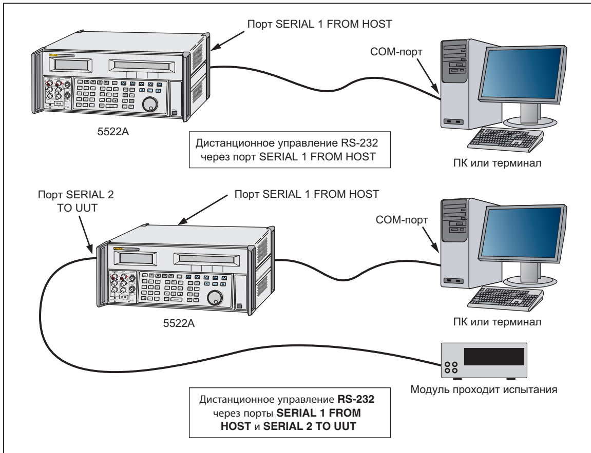
Рис. 1-2. Дистанционные соединения RS-232
