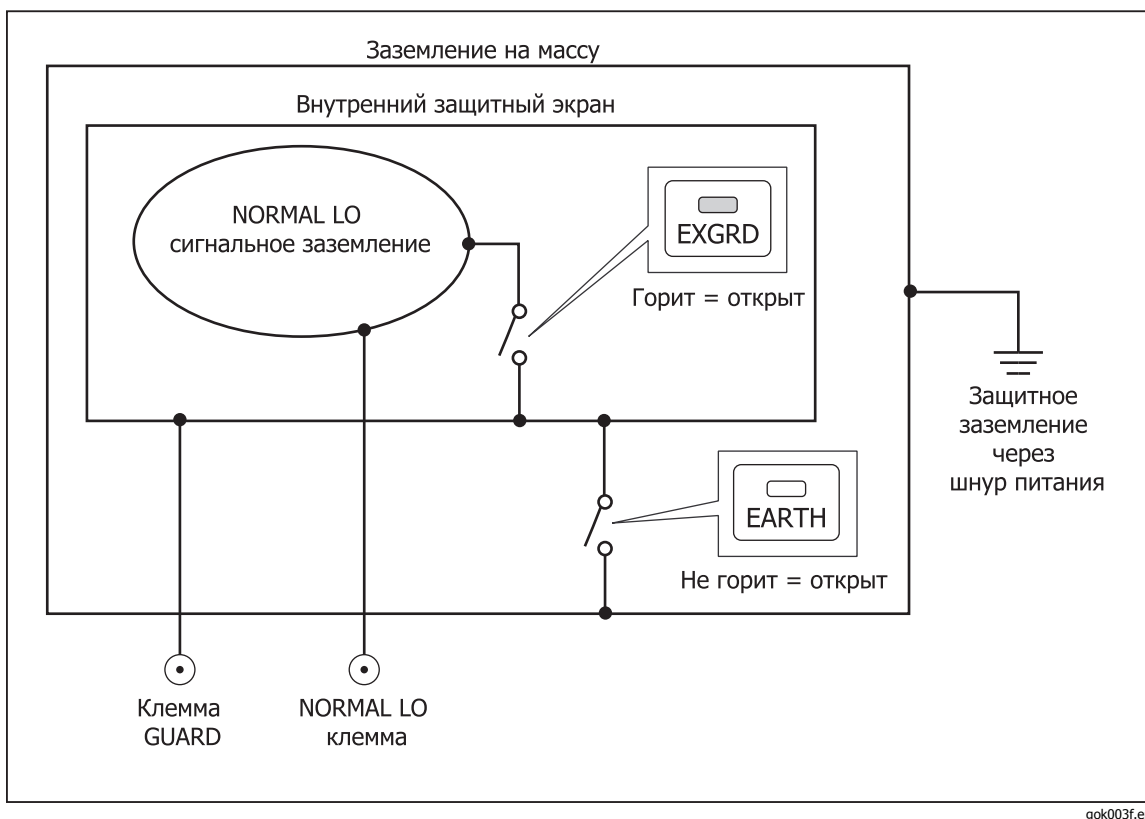
Рисунок 4-1. Внутренние соединения EARTH и EXGRD
