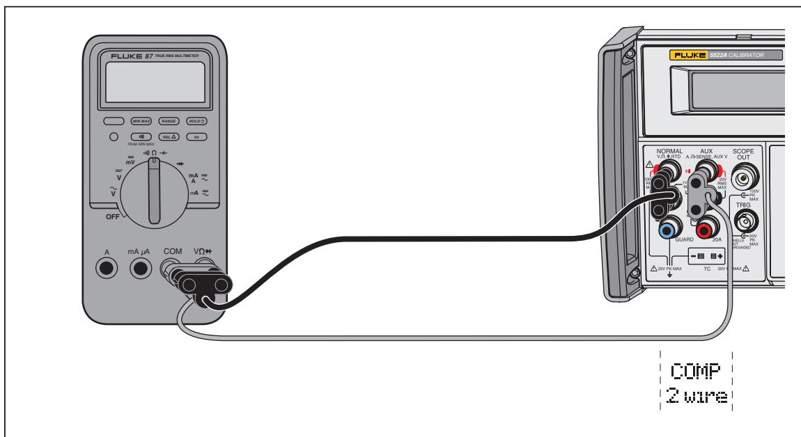
Рисунок 4-5. Подключение испытываемого устройства: Емкость (2-проводная компенсация) gjh017.eps
