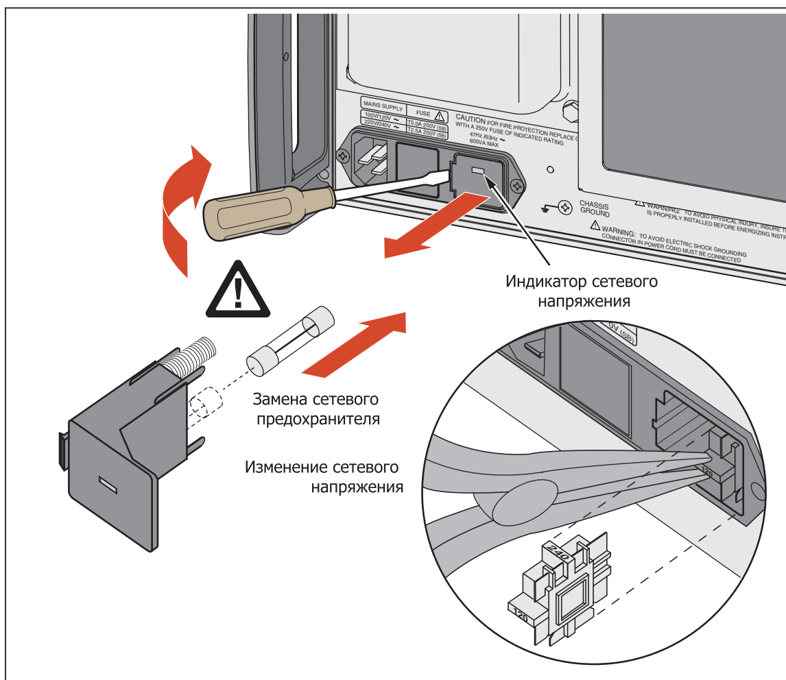
Рисунок 7-1. Извлечение предохранителя
