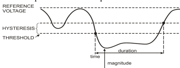
Рис. Характеристики события напряжения – «Провал» / voltage dip
