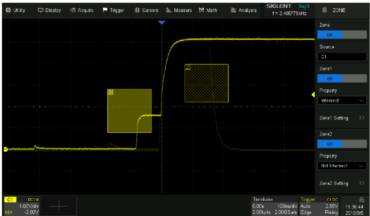
Рис. 18-5 Синхронизация по заданной области
