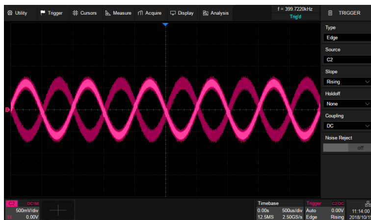
Рис. 18-1 Функция подавления шума отключена
