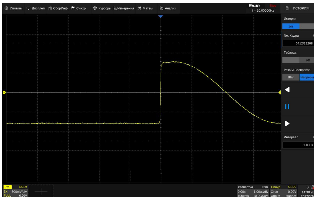
Рис. 16-1 Вывод 5412-го кадра, сегментированной памяти в режиме истории
