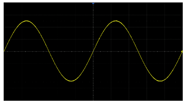
ERES (3 бита)
