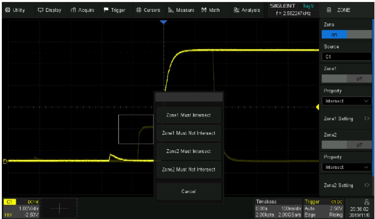
Рис. 18-4 Пример выделения области синхронизации
