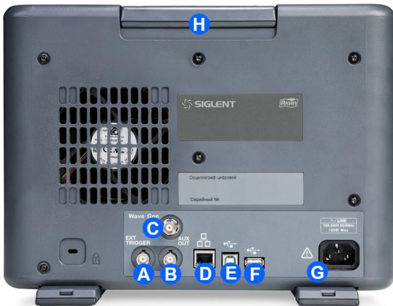
Рис. 9-2 Задняя панель осциллографов серии АКІП-4140
