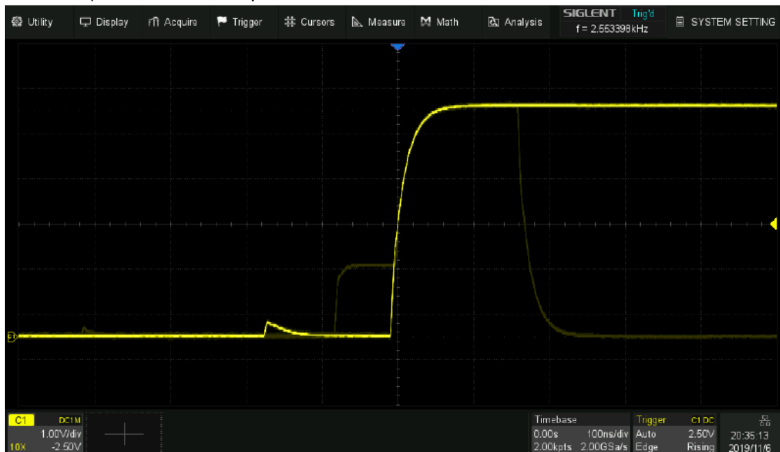
Рис. 18-3 Отображение аномалии в режиме послесвечения
