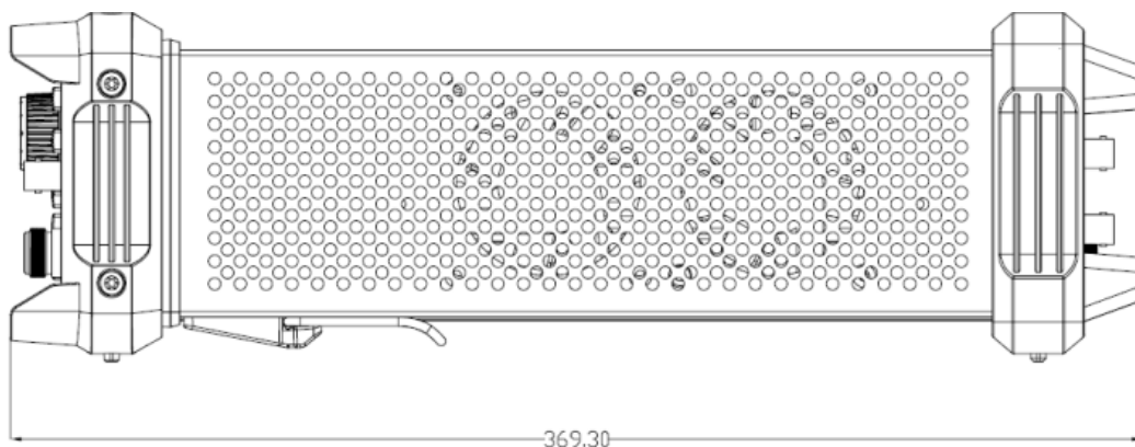
Рис 2-3 Вид сбоку
