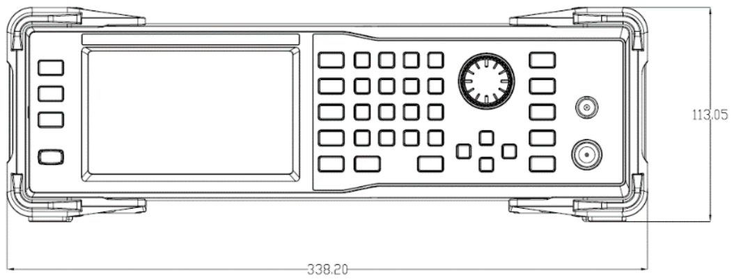
Рис 2-1 Вид спереди
