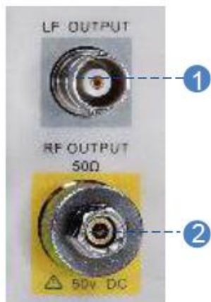
Рис 5-3 Разъемы передней панели
