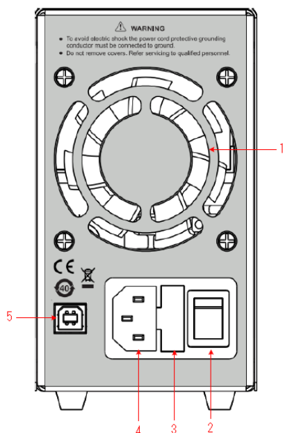
Рис. 5.2 Задняя панель
